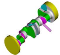
Bearbeitungssimulation einer Kurbelwelle aus dem Vollen im Volumenmodell
